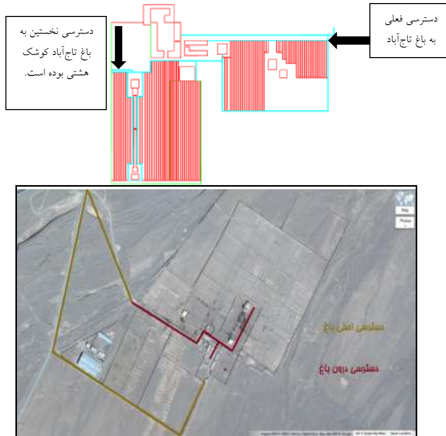
شکل ۴: دسترسى‌هاى اصلى و فرعى (درون باغ) فعلى باغ (نگارندگان)
