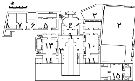
نقشه ۲: معرفی فضاهای موجود در بنای حوضخانه همایون فال (نگارنده)
