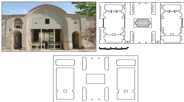
شکل ۱۷: شکل و مدل ساده گرافیکی پلان حوضخانه مزرعه مبارک‌آباد
