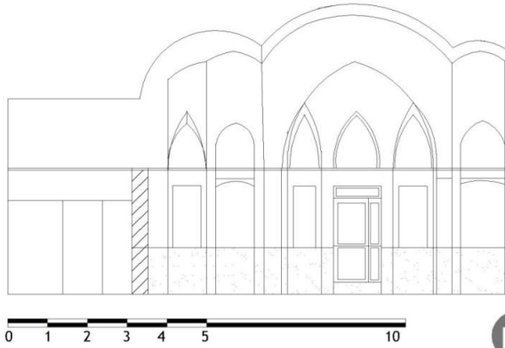
برش A-A خانه باغ لاجوردی (تعظیمی فر)
