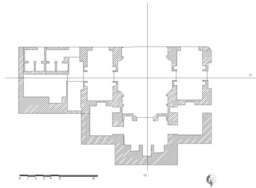
پلان عمارت لاجوردی (تعظیمی فر)
