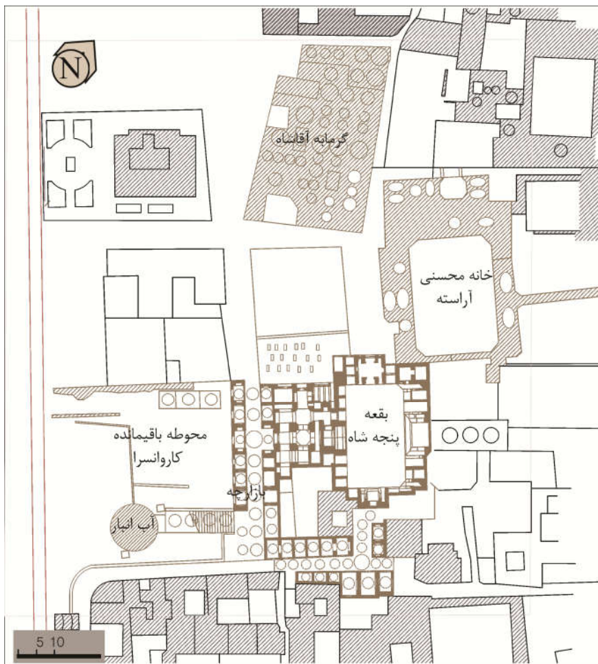
تصویر (۳۳): نقشه بازسازی وضعیت مرکز محله پنجه‌شاه و حجره‌های بازارچه در سال ۱۳۳۵ (نگارندگان)
