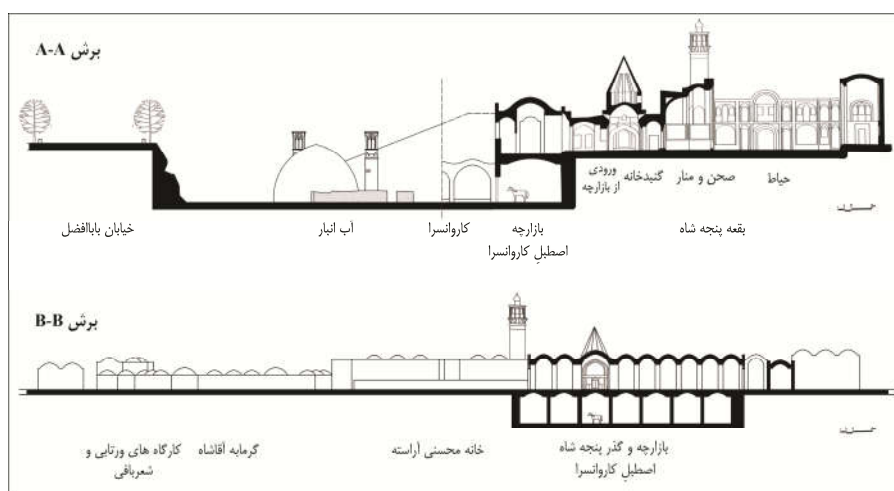
تصویر (۳۲): بازسازی برش‌های وضعیت مرکز محله و عناصر اطراف در سال ۱۳۳۵ (نگارندگان)
