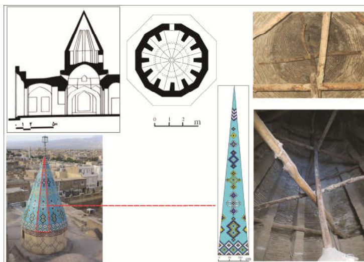
تصویر (۸): وضعیت موجود پلان، تزیینات و برش و نمای داخل گنبد رک بقعه (نگارندگان)
