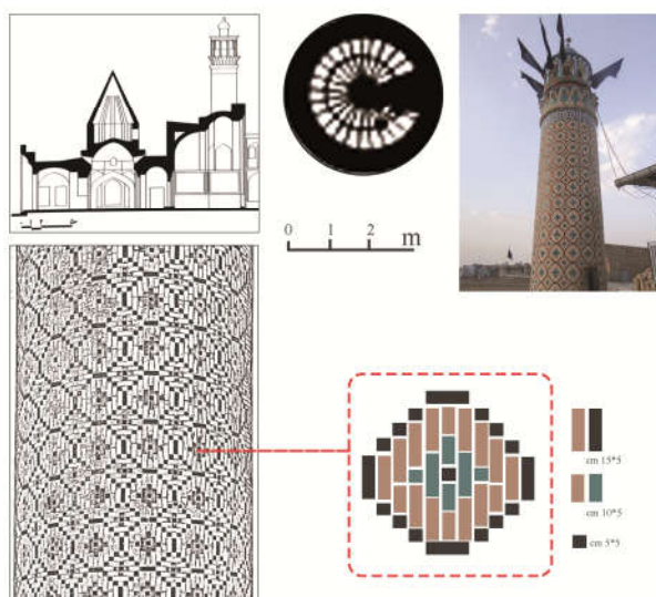
تصویر (۹): وضعیت موجود پلان، تزیینات و نمای منار بقعه (نگارندگان)
