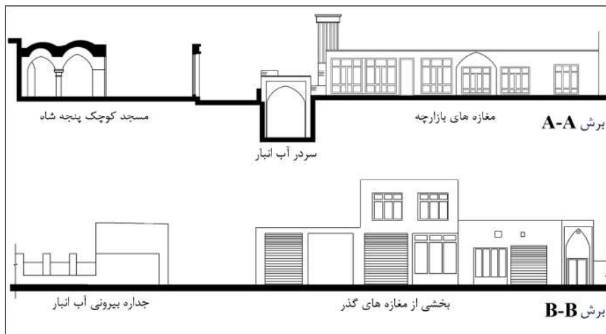
تصویر (۱۱): مقطع - نماهای وضعیت فعلی مجموعه پنجه شاه و حجره های باقی مانده (نگارندگان: بر اساس نقشه های مندرج در پرونده ثبت)
